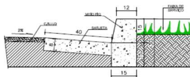
CORTE ESQUEMÁTICO DO MEIO FIO C/ SARJETA
