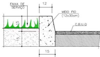
CORTE ESQUEMÁTICO DO MEIO FIO
